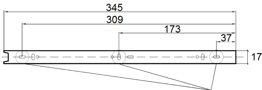
Монтажные отверстия, используемые для крепежа
