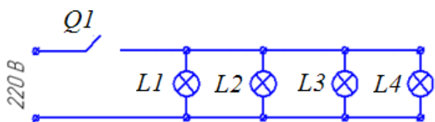
Схема электрическая
