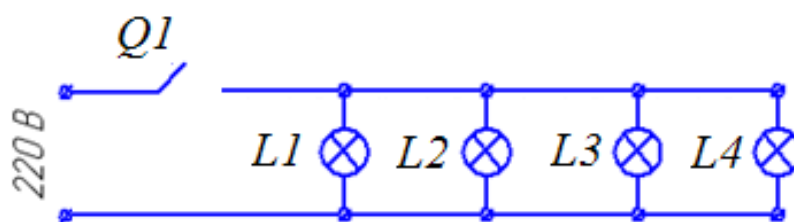
Схема электрическая
