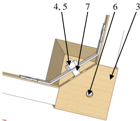
Рисунок 1 – Схема крепления ноги
