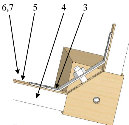
Рис. 1. Схема крепления ноги
