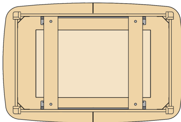
Рис.3 Схема хранения вставки
