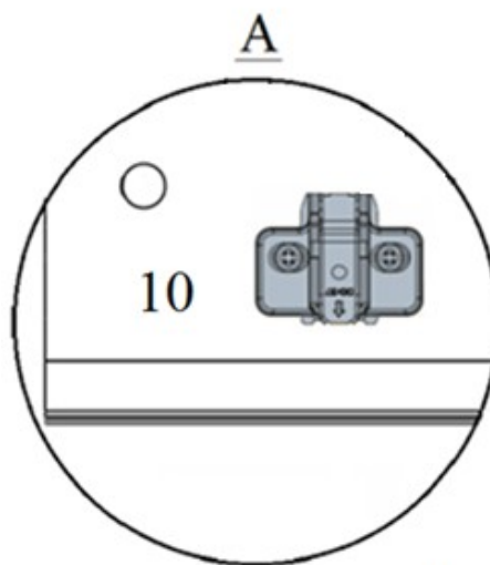
установка ответной планки петли
